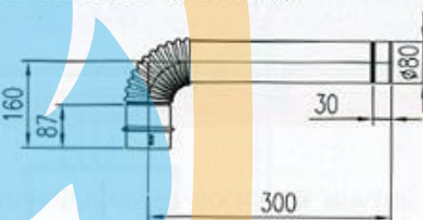
DGB-EL90 (Угол 90°)
