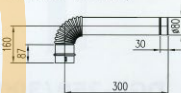
DGB-EL90 (Угол 90°)
